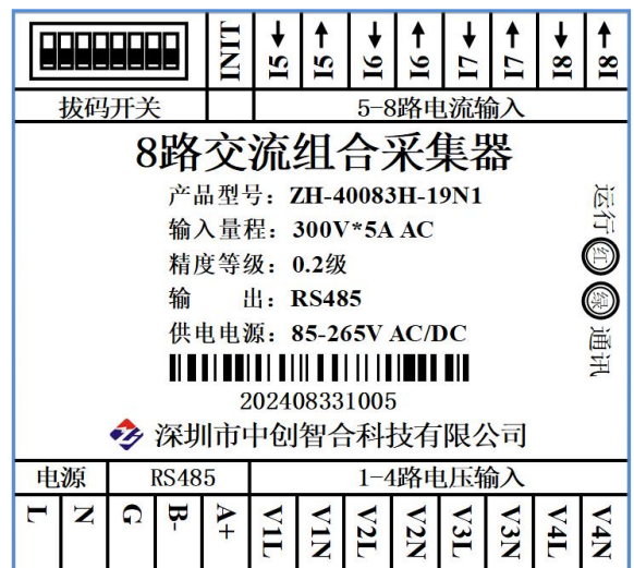
图 4.6、组合型定义图(可指定任意组合,RS485 接口)
