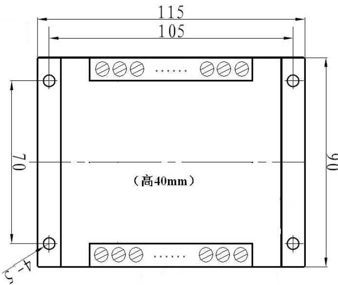
图 4.3、产品尺寸图（高：40 mm）
